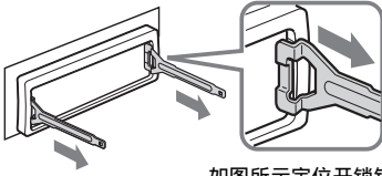
如图所示定位开锁钥匙。
